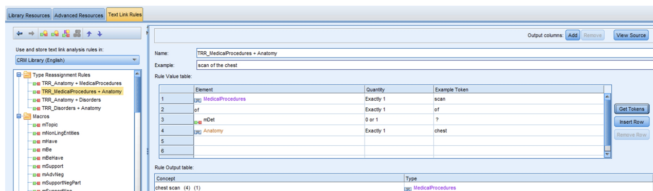
Figura 36. TRR para procedimientos médicos + anatomía
