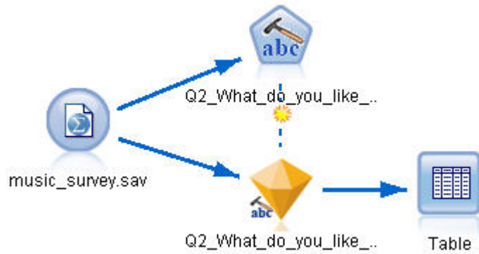
Figura 3. Ruta de ejemplo: Nodo de archivo de estadísticas con un nugget de modelo de concepto de minería de textos
