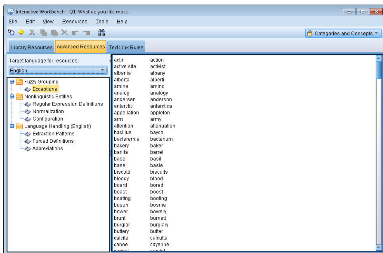
Figura 42. Editor de plantillas de minería de textos: pestaña Recursos avanzados
