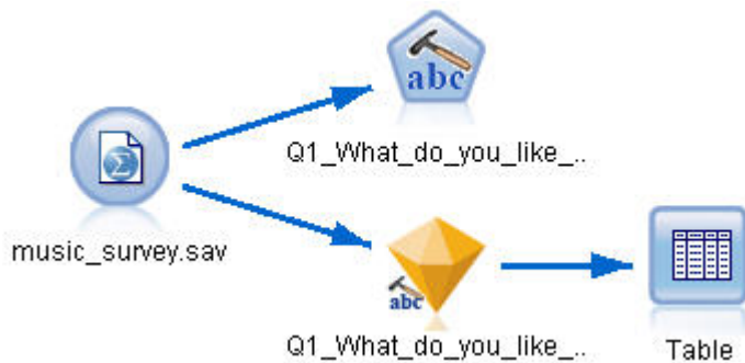
Figura 9. Ruta de ejemplo: Nodo de archivo de estadísticas con un nugget de modelo de categoría de minería de textos
