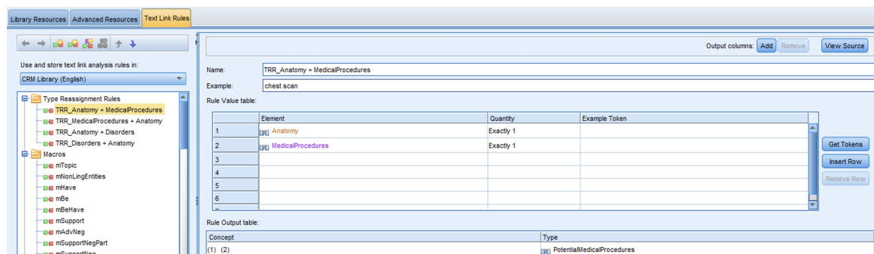
Figura 35. TRR para anatomía + procedimientos médicos
